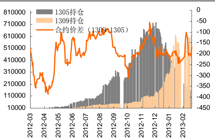
图3-10: 9月5月价差为28
