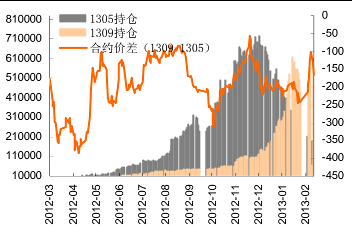
图3-10: 9月5月价差为-13
