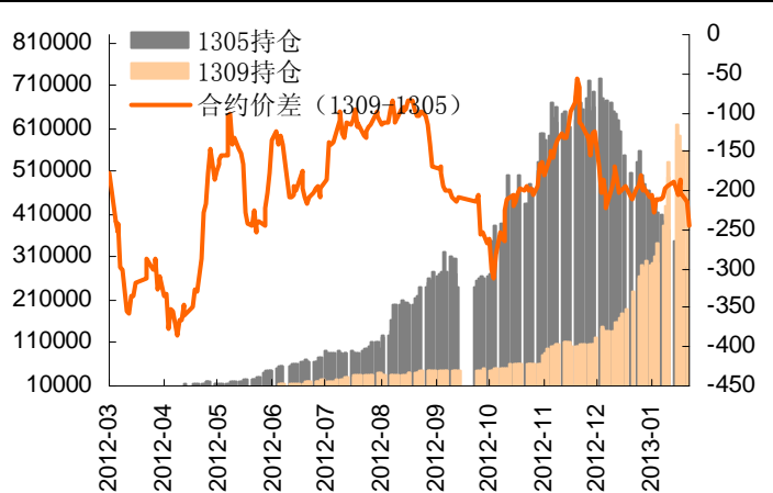
图3-10: 9月5月价差为47
