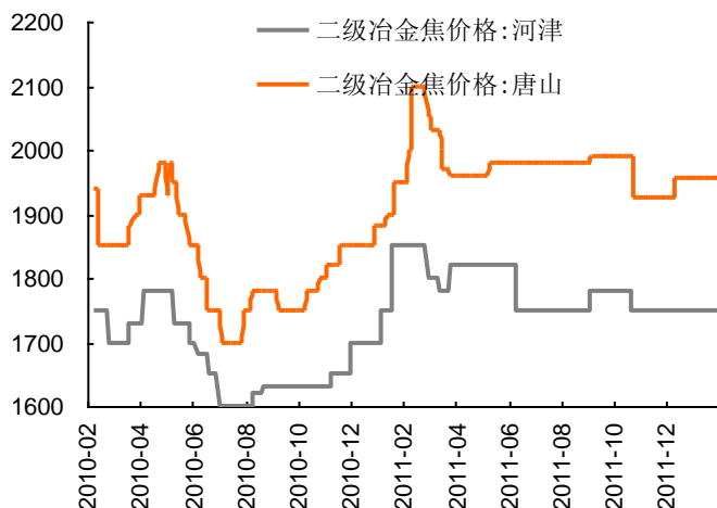
图4-9: 原材料冶金焦价格变动
