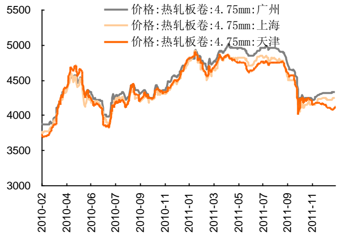
图4-6: 主要城市热轧板卷4.75mm价格
