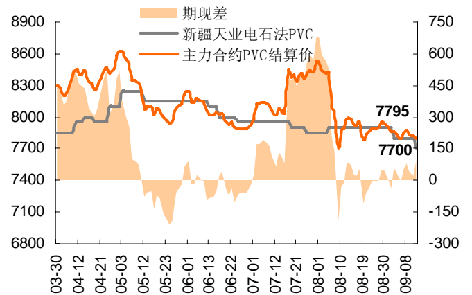
图2-6: PVC期现价格走势图
