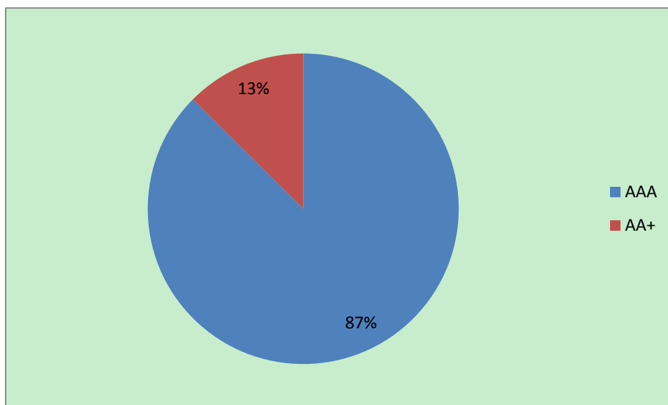
图 3：平安财富-周成长（净值型）2015 年 1 期人民币理财产品
